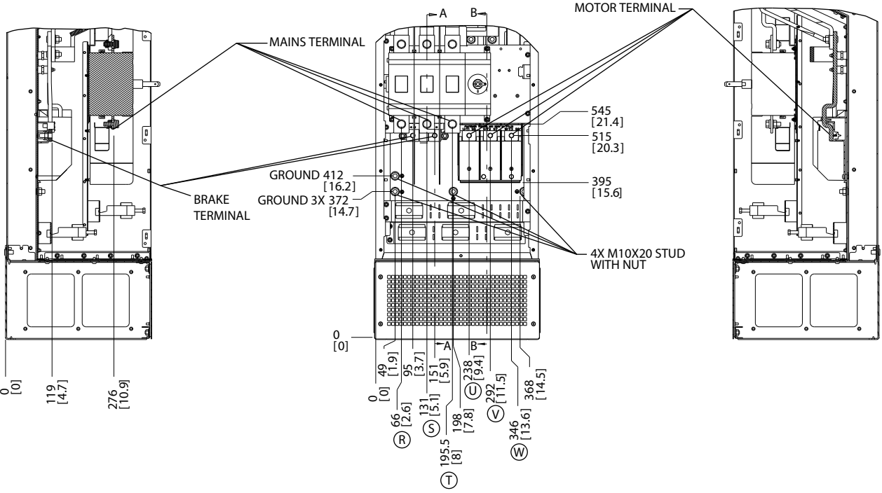
Çizim 2.18 Terminal Yerleri, Bağlantı Kesme Anahtarlı Seçeneği ile D7h
