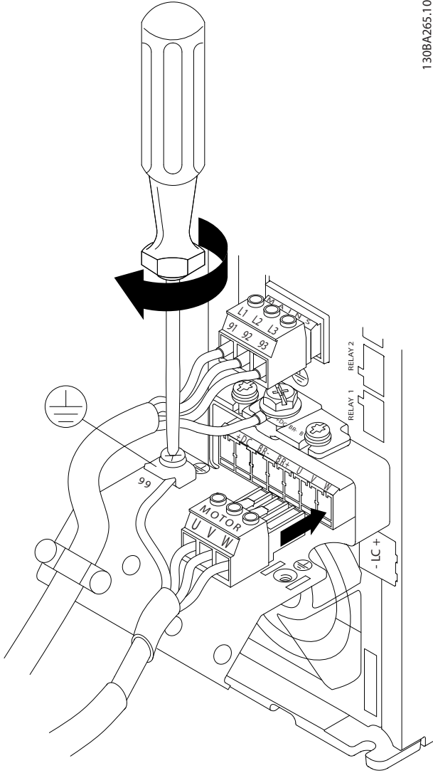
Çizim 2.11 A2 ve A3 için motor bağlantısı
