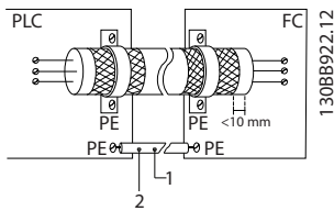
Çizim 2.22 Doğru blendajlama
